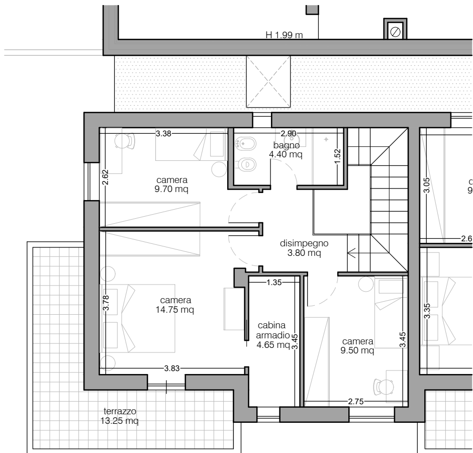
PIANO PRIMO scala 1:100
